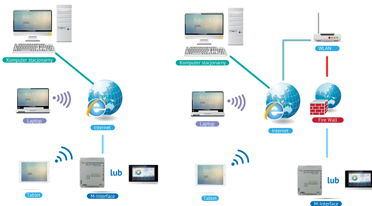
Sieć LAN
